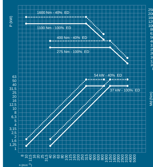
Main spindle - left 54(37) kW - 3300 min -1
