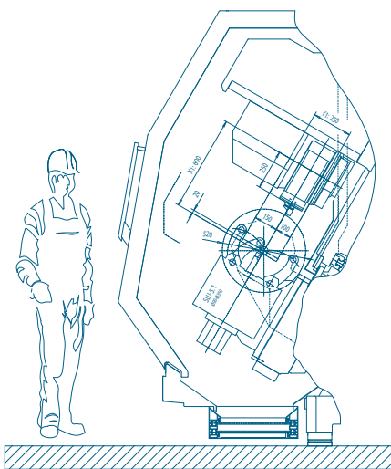
M30 | M35 MILLTURN
