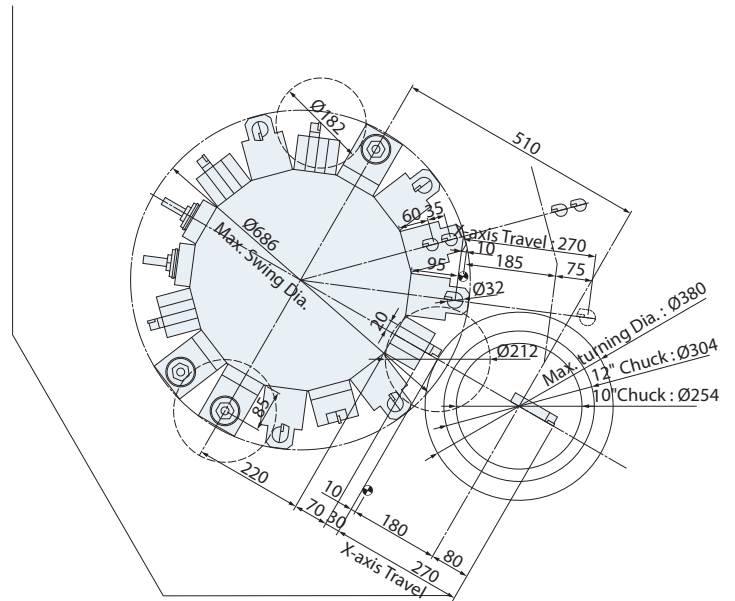
【 Y-axis model 】 ▶ 90° Live tool
